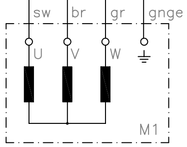
Sternverschlaltung
