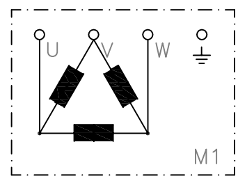
Dreieckverschlaltung
