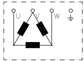
Dreieckverschaltung
