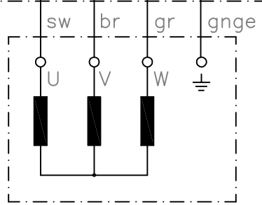
Sternverschaltung
