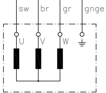
Sternverschaltung
