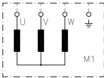
Sternverschaltung
