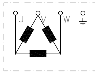
Dreieckverschaltung
