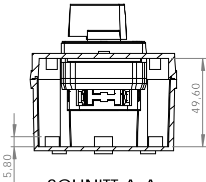
SCHNITT A-A
