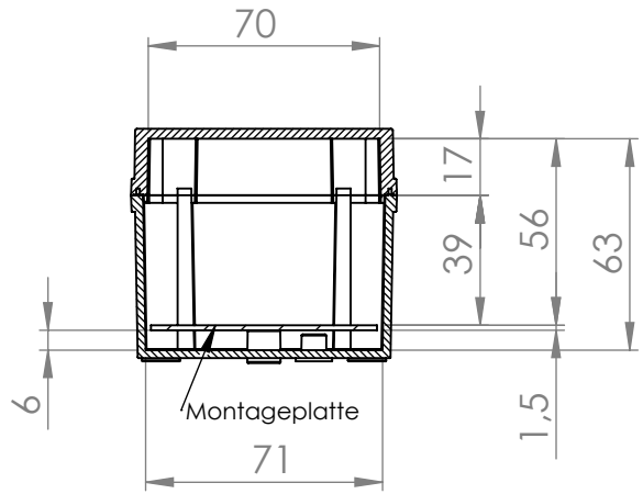
Innenansicht Oberteil
