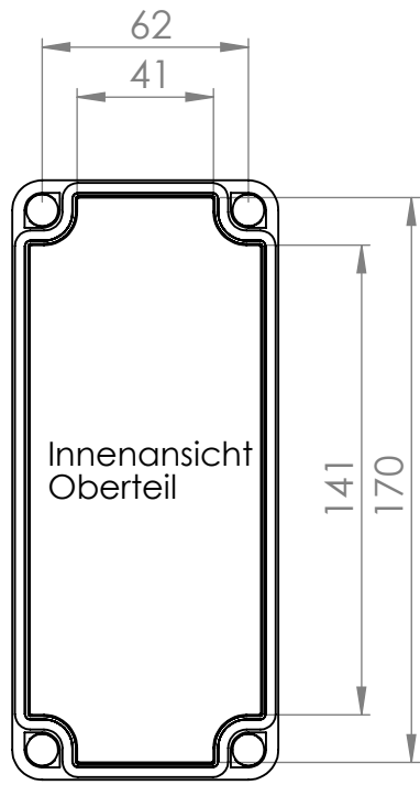
Innenansicht Oberteil
