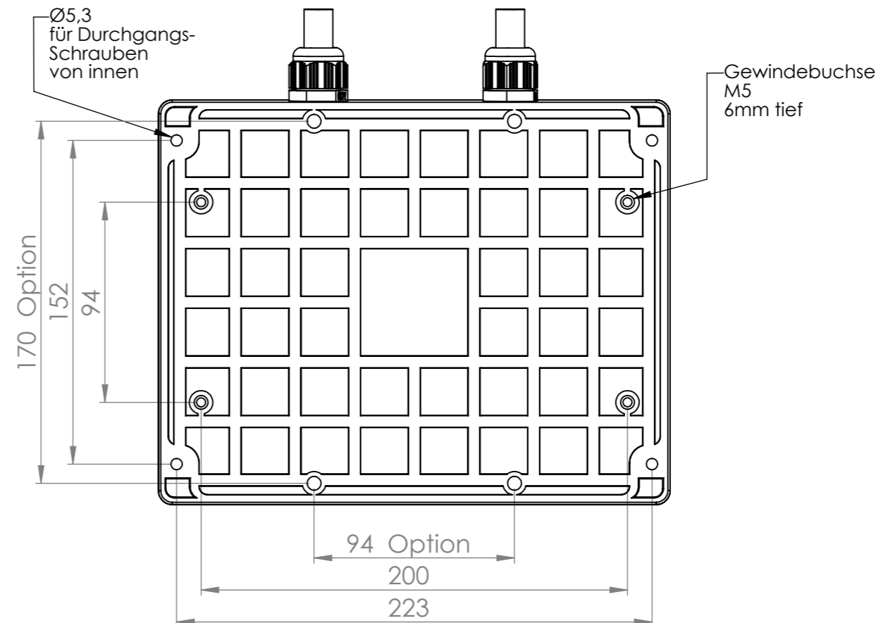
Ansicht "A"
