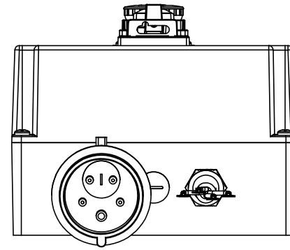
Phasenwender
