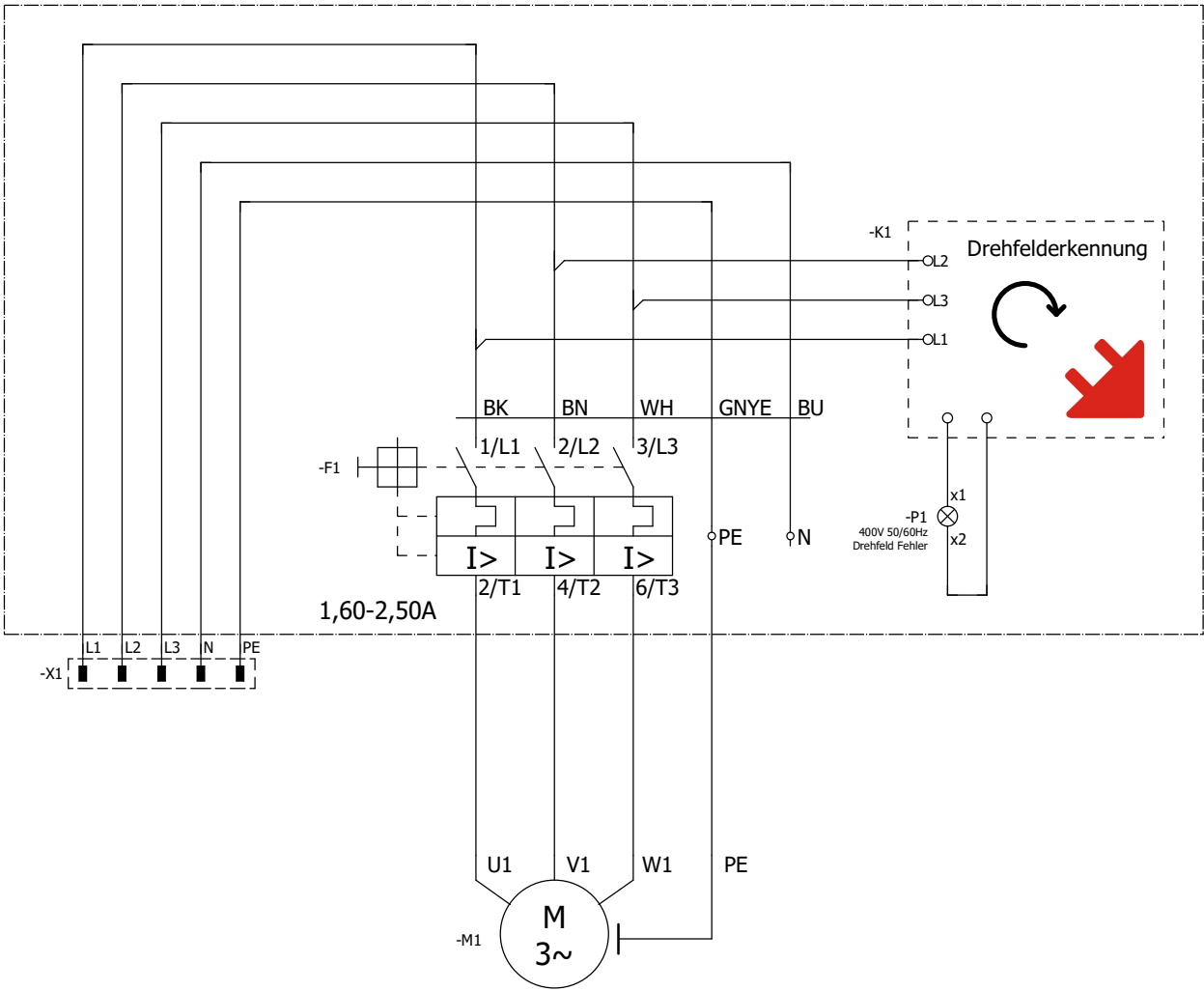
Einspeisung
