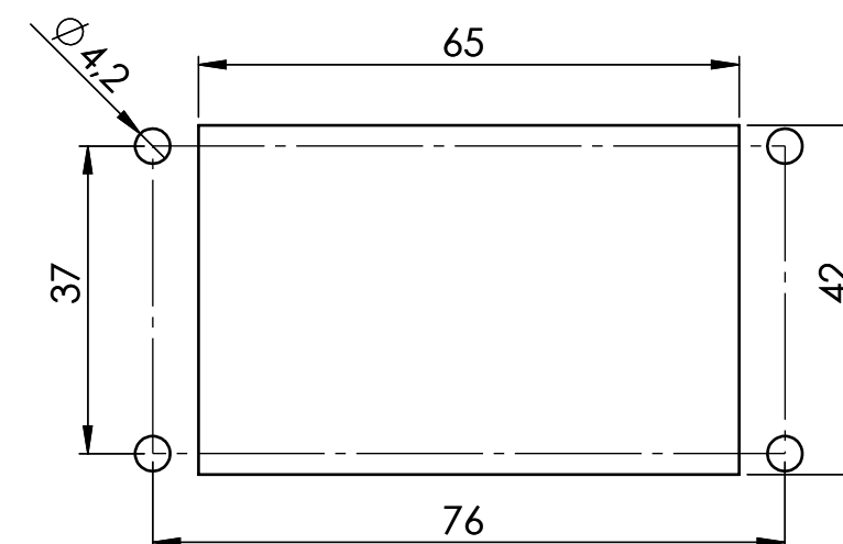
Einbaumaße
