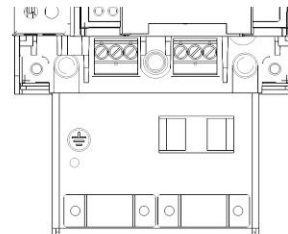
Kabelfäste för matning- samt motorkabel
