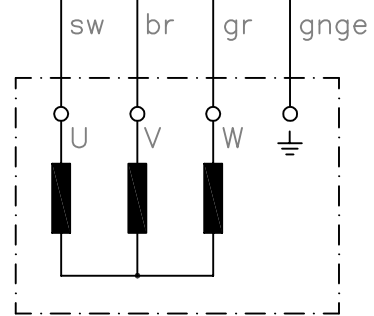
Sternverschaltung
