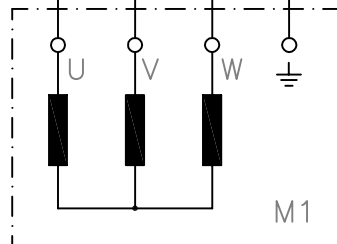
Sternverschaltung
