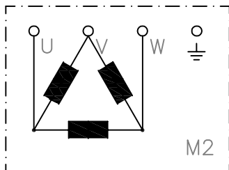
Dreieckverschaltung
