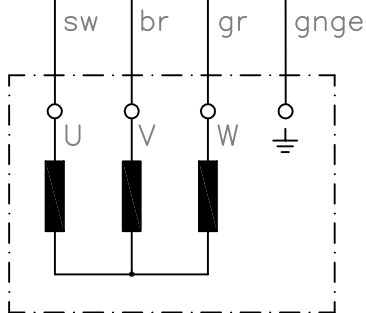
Sternverschaltung
