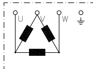
Dreieckverschlaltung
