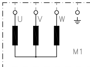
Sternverschlaltung
