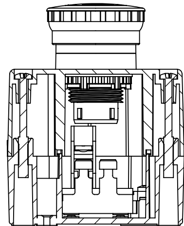
SCHNITT A-A
