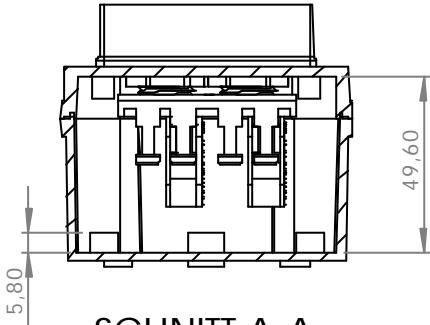
SCHNITT A-A
