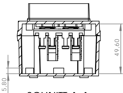
SCHNITT A-A
