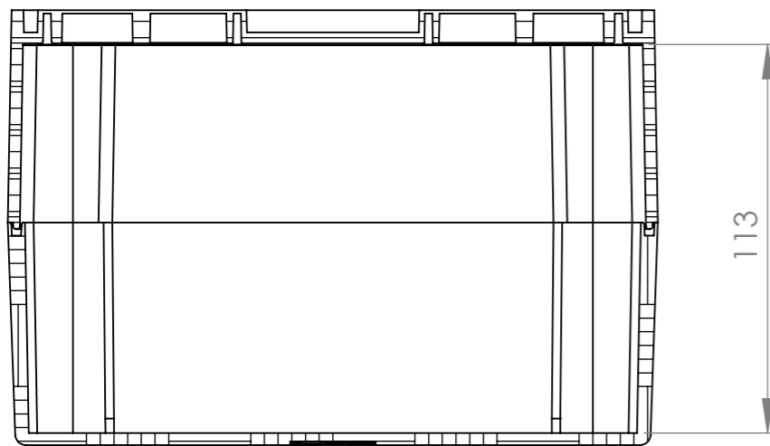
SCHNITT A-A
