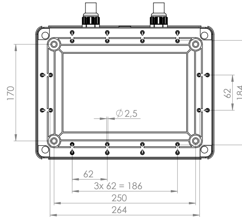
Ansicht "A"
