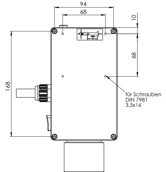
Ansicht "A"
